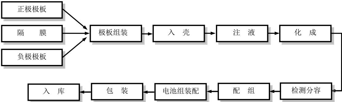
3、电池组装工艺流程图
