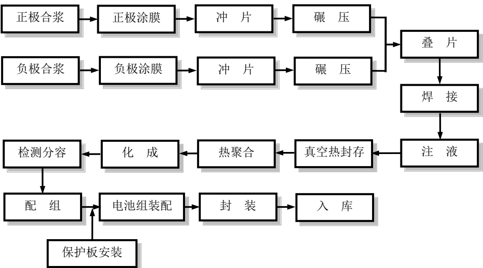
2、镍系电池生产工艺流程图
