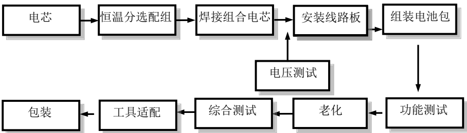
4、电源管理系统（BMS）生产工艺流程图
