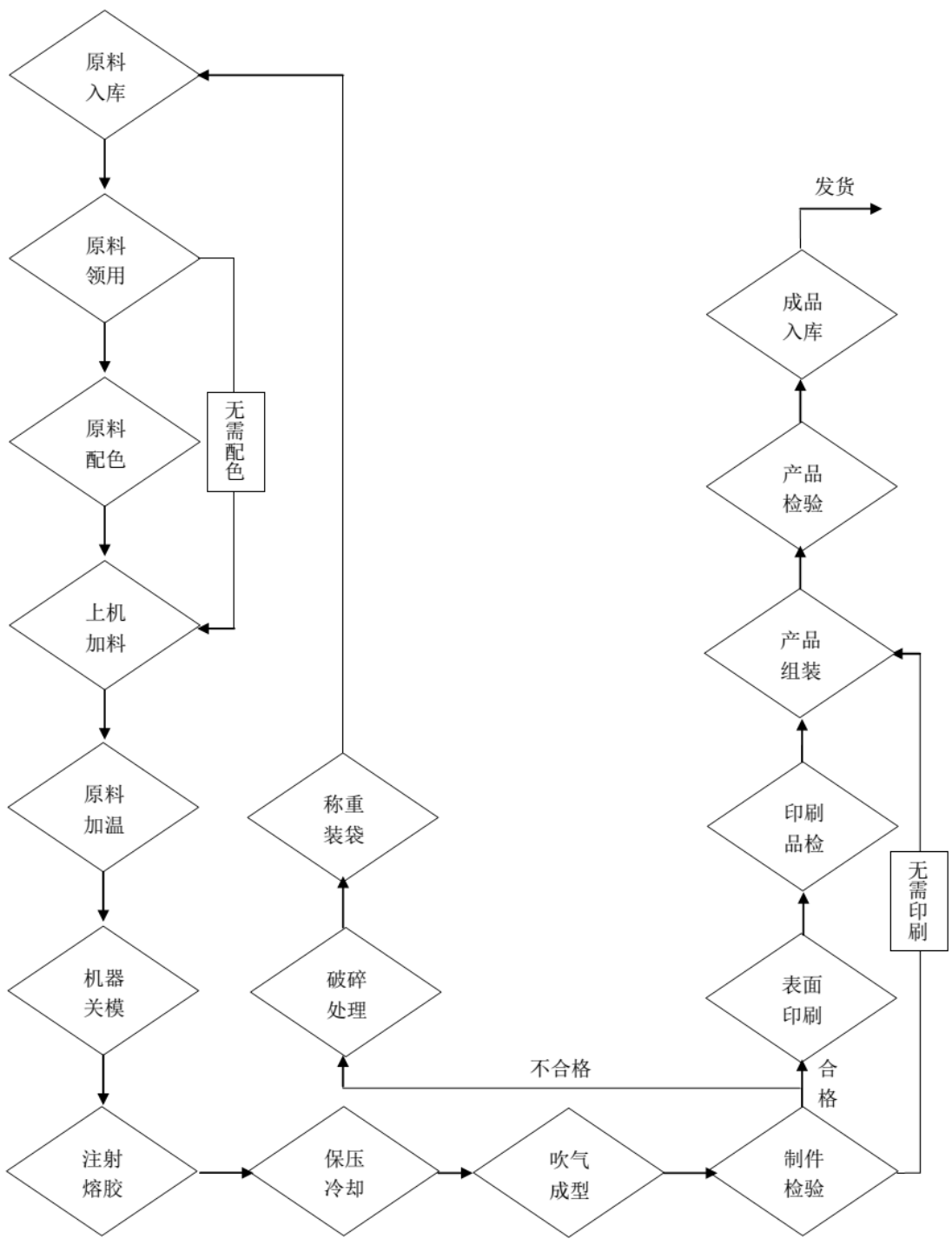
②奶嘴生产流程
