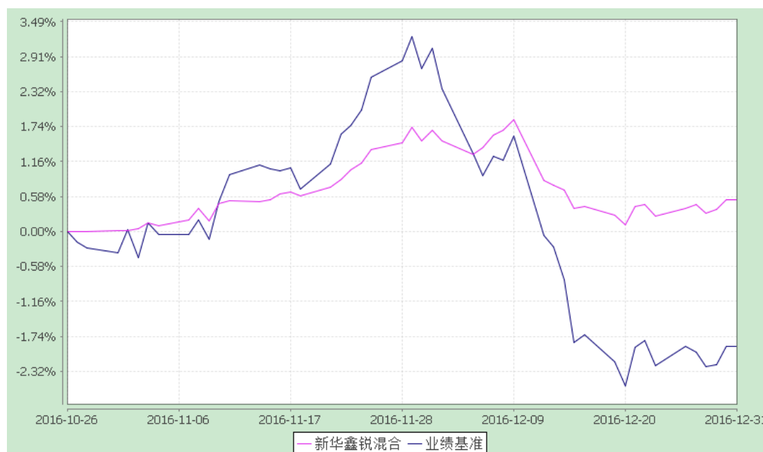
新华鑫锐混合型证券投资基金 累计净值增长率与业绩比较基准收益率历史走势对比图 (2016 年 10 月 26 日至 2016 年 12 月 31 日)
