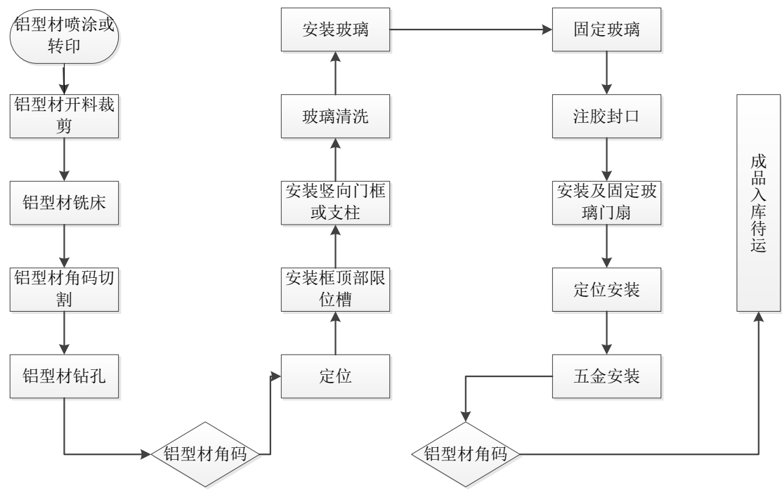
铝合金门窗幕墙生产工艺流程图
