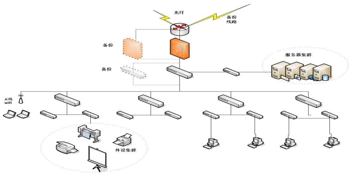
信息化系统网络拓扑图
