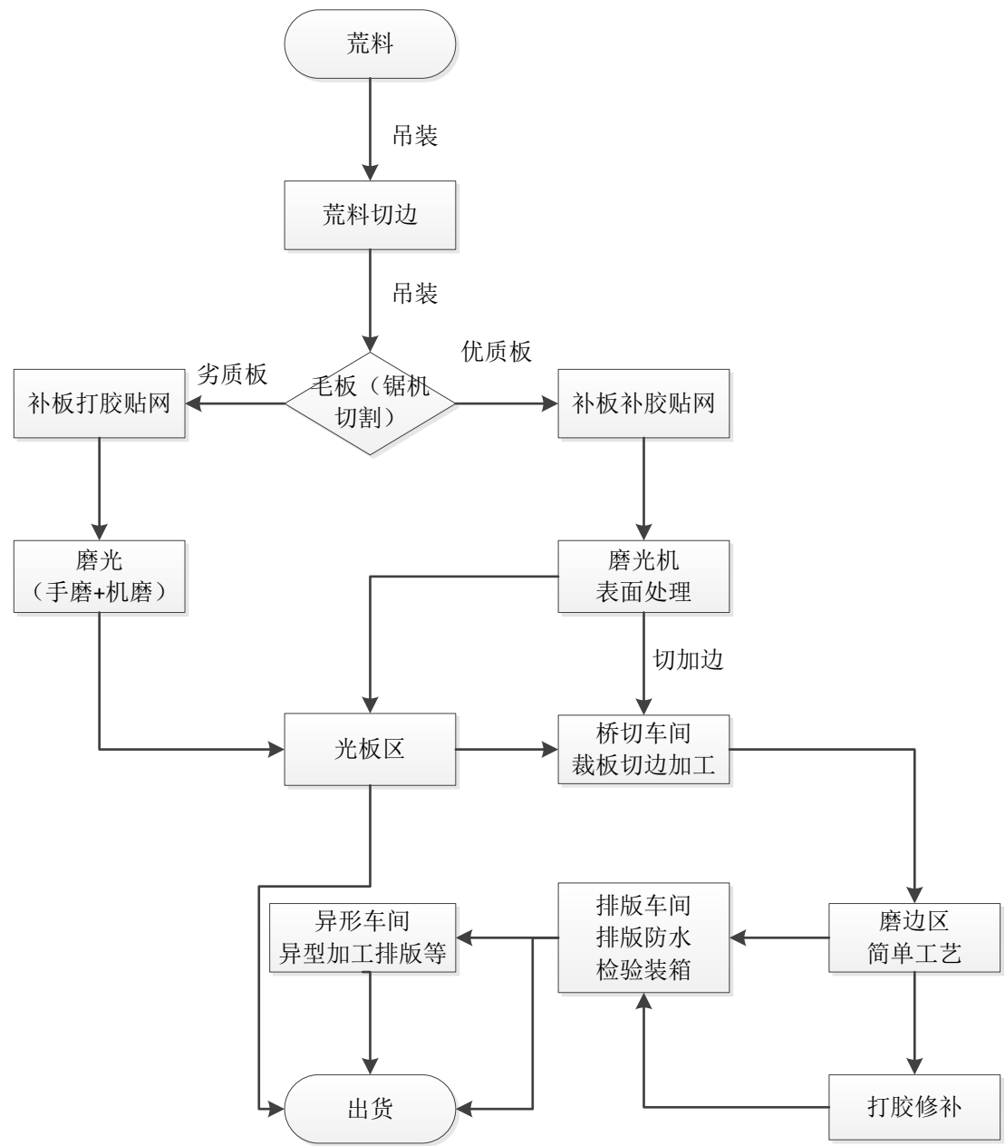
复合型石材制作工艺流程图
