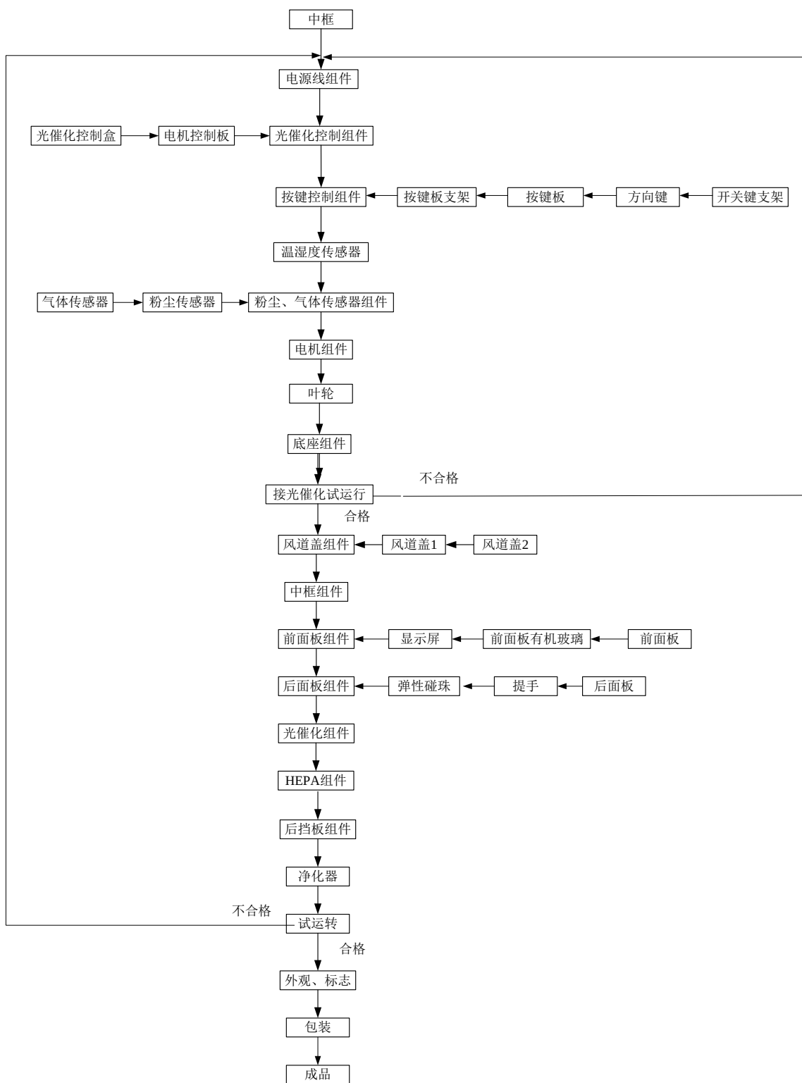
(2) 尾气净化装置流程图
