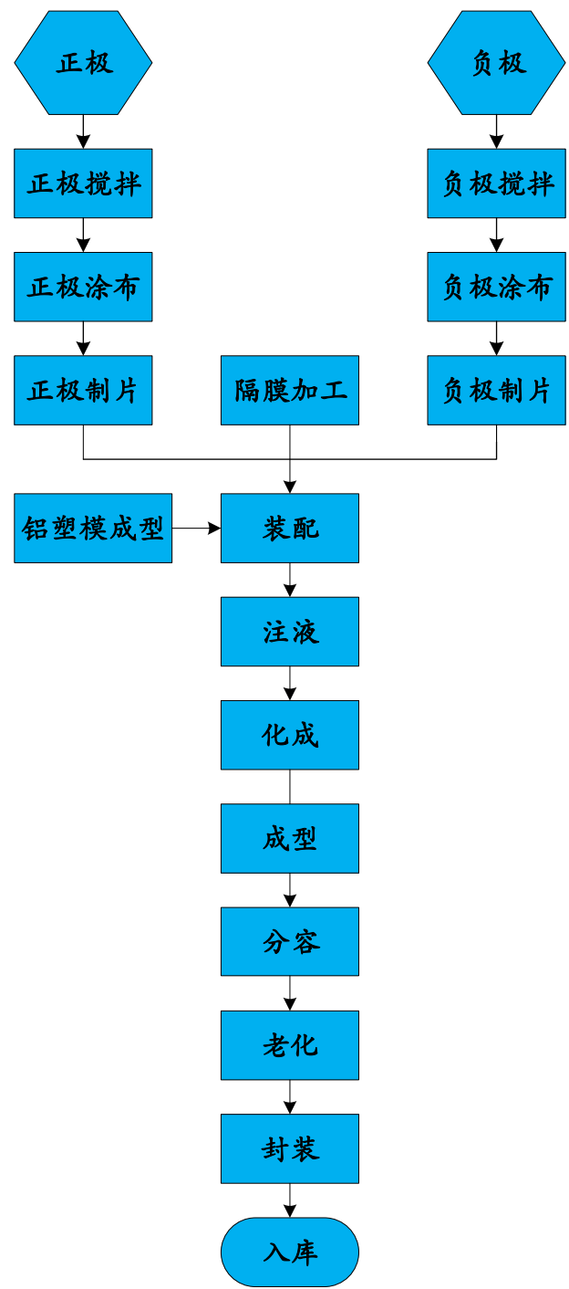
(2) 铝壳类锂离子电池制造流程图
