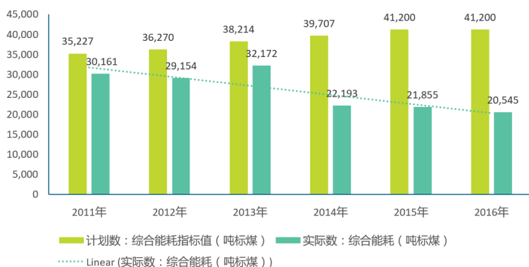
2011-2016年综合能耗使用量
