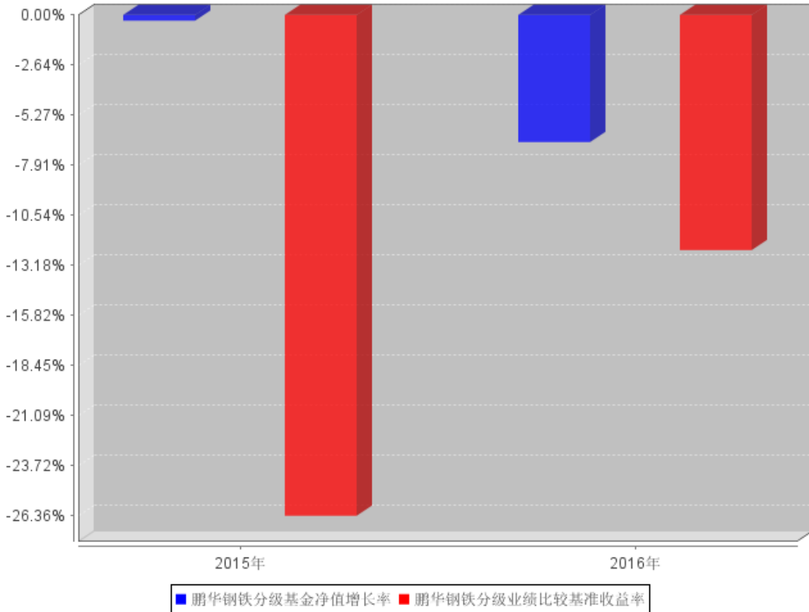
鹏华钢铁分级自基金合同生效以来基金每年净值增长率及其与同期业绩比较基准收益率的对比图
