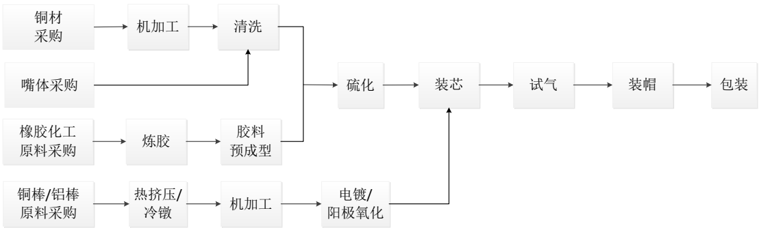
①气门嘴工艺流程图
