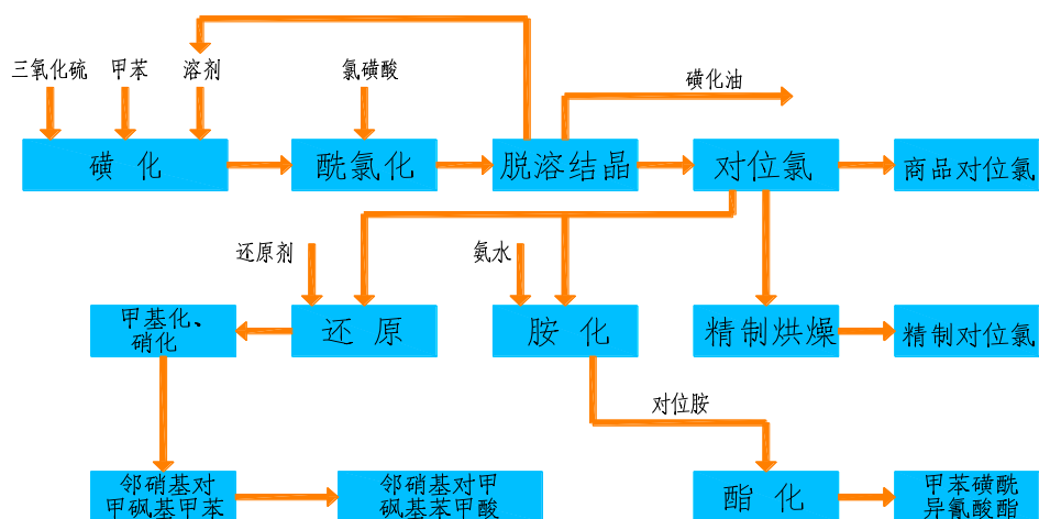
新材料装置流程框图
