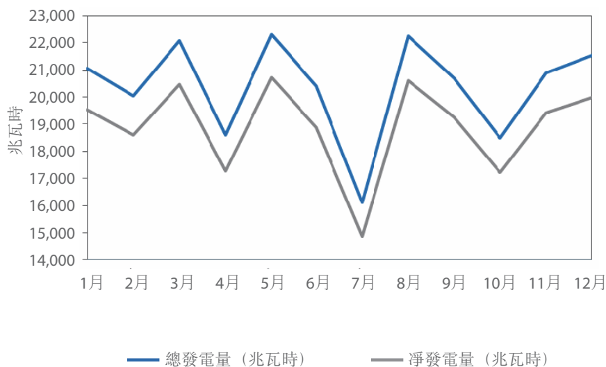
圖2.3碭山發電量 — 2016年
