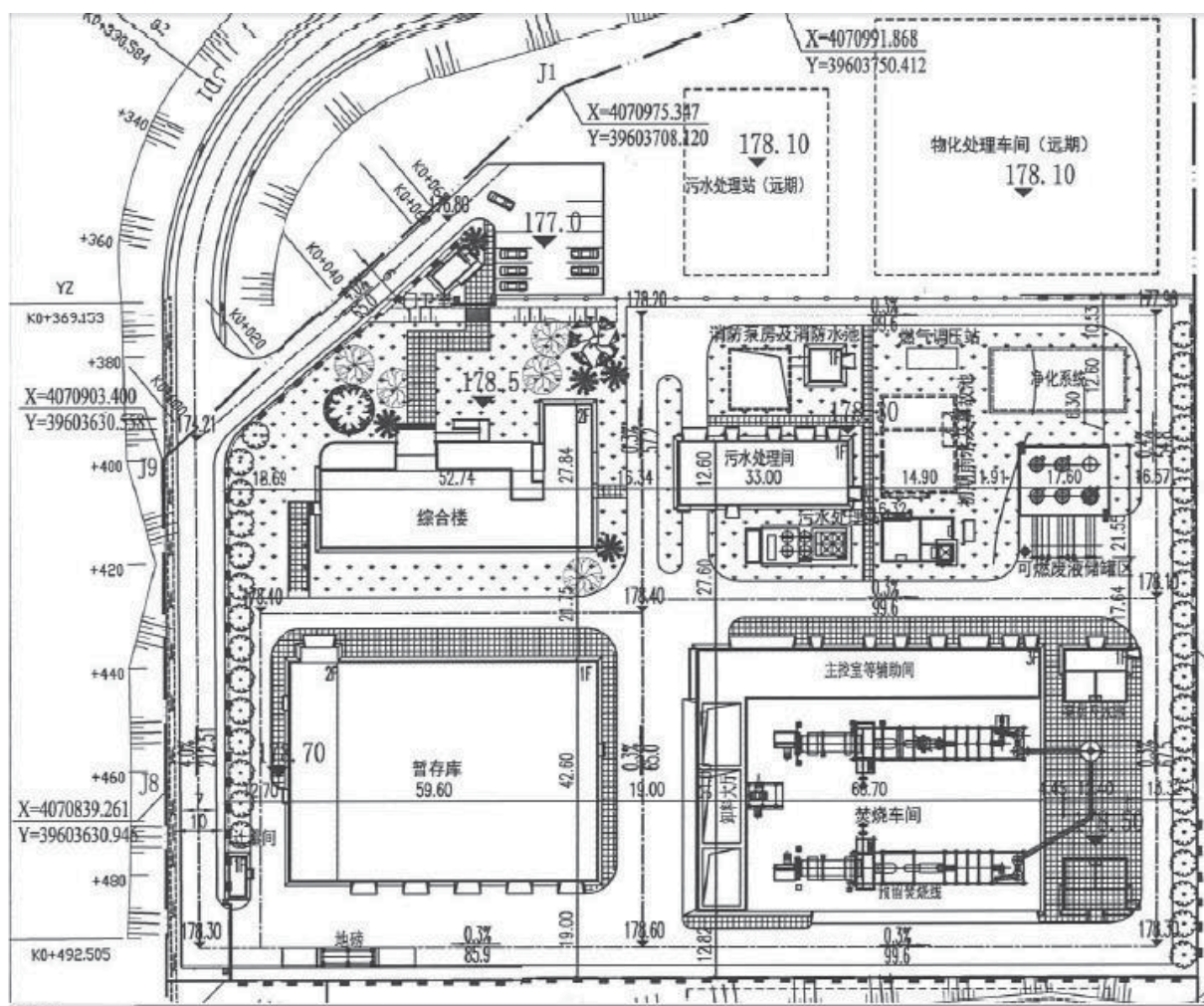
圖4.1淄博危廢平面佈置圖
