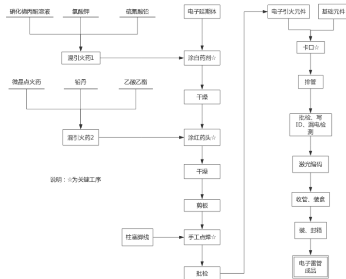
图 5 电子雷管生产工艺流程框图
