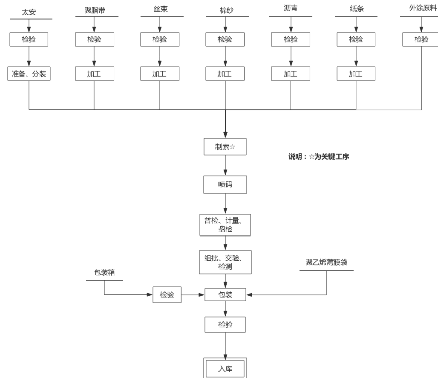
图7 导爆索生产工艺流程框图
