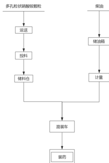
图9 多孔粒铵油炸药工艺流程图
