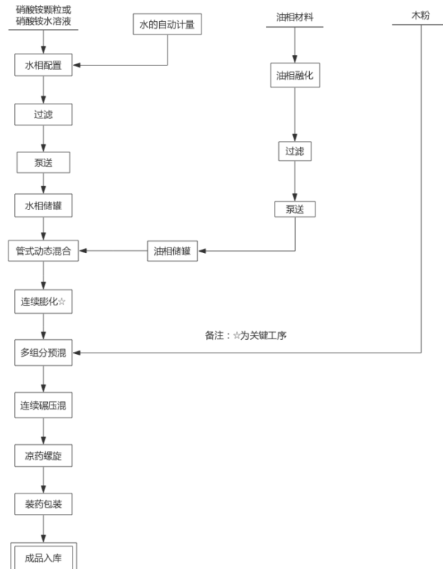
图 1 膨化硝铵炸药生产工艺流程图
