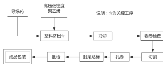
图 6 导爆管生产工艺流程框图
