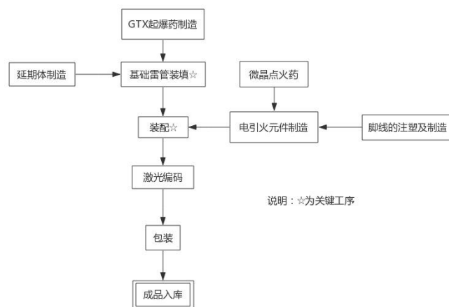
图 3 工业电雷管生产工艺流程图
