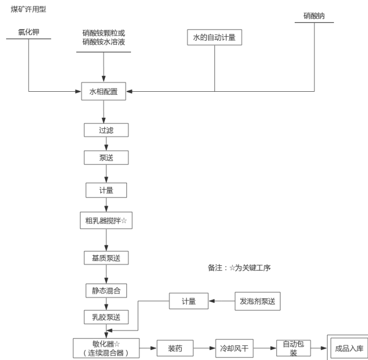
图 2 乳化炸药生产工艺流程图
