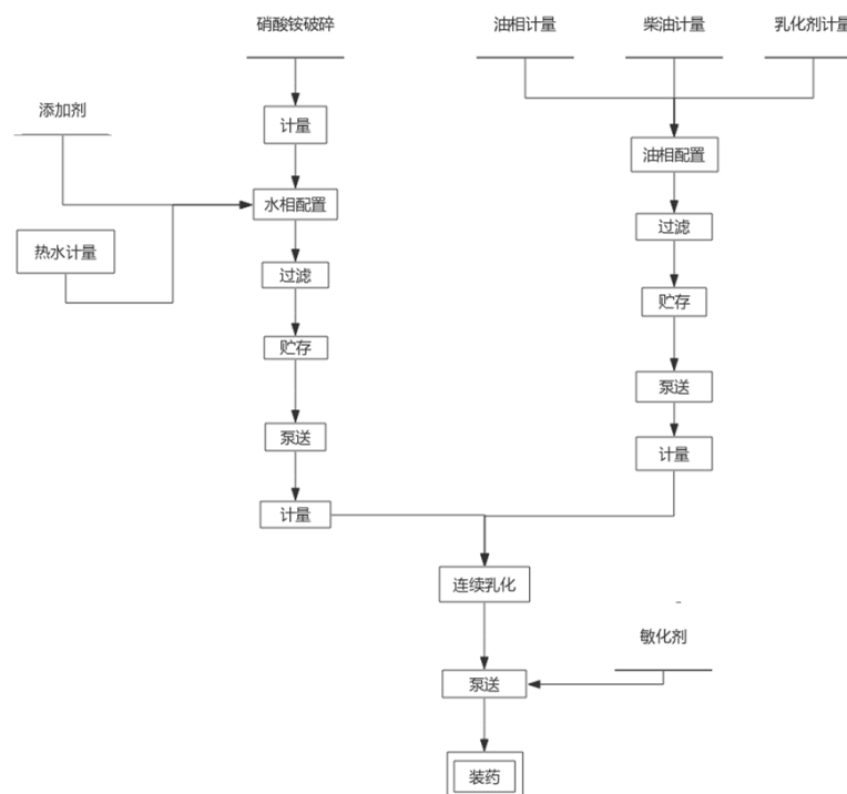
图8 现场混装乳化炸药（地面站制乳）工艺流程图
