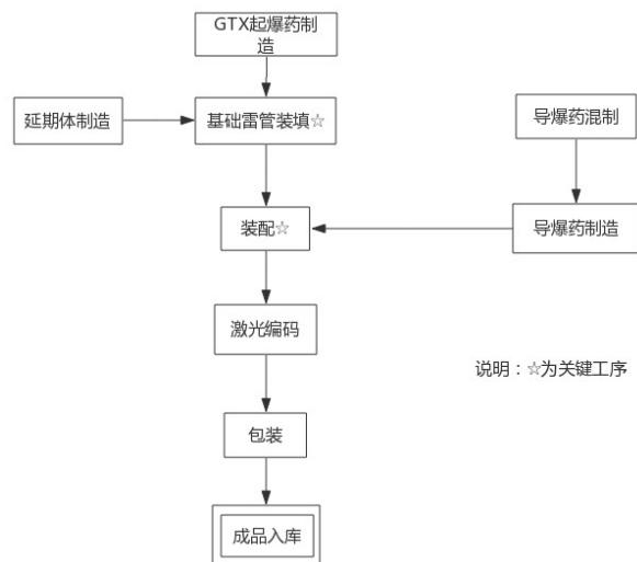
图 4 导爆管雷管生产工艺流程框图
