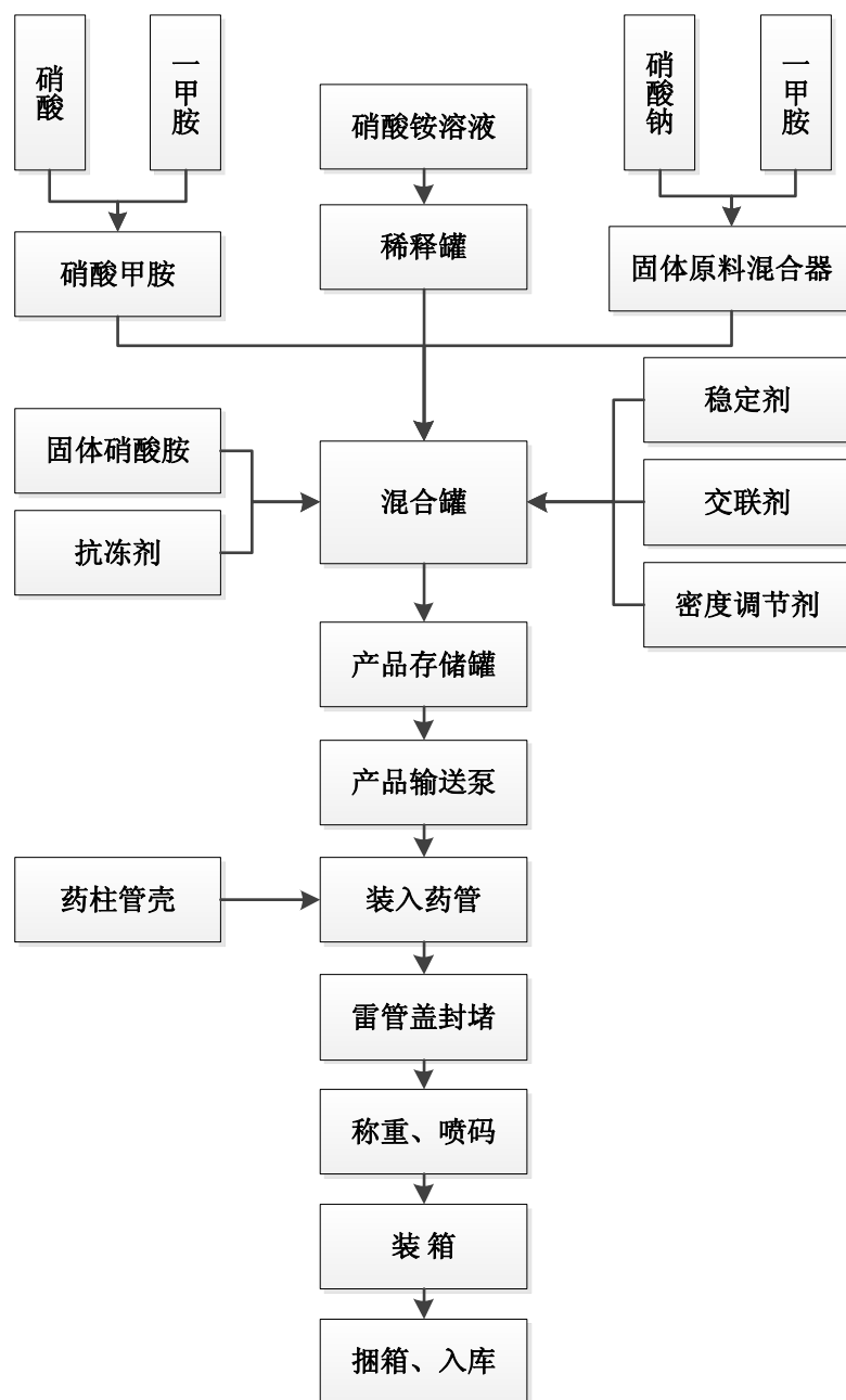
⑤工业电雷管工艺流程图
