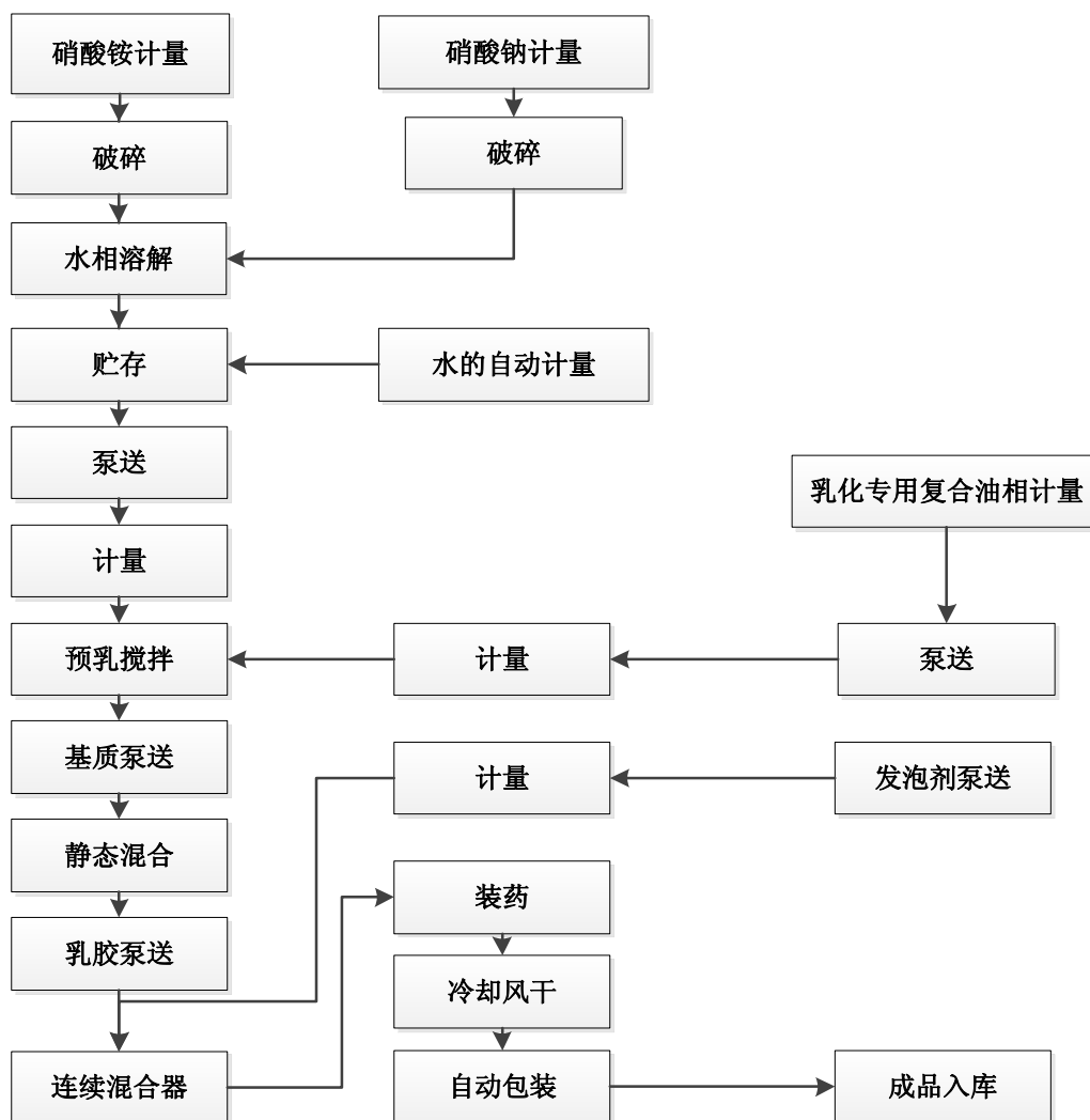
②现场混装炸药工艺流程图
