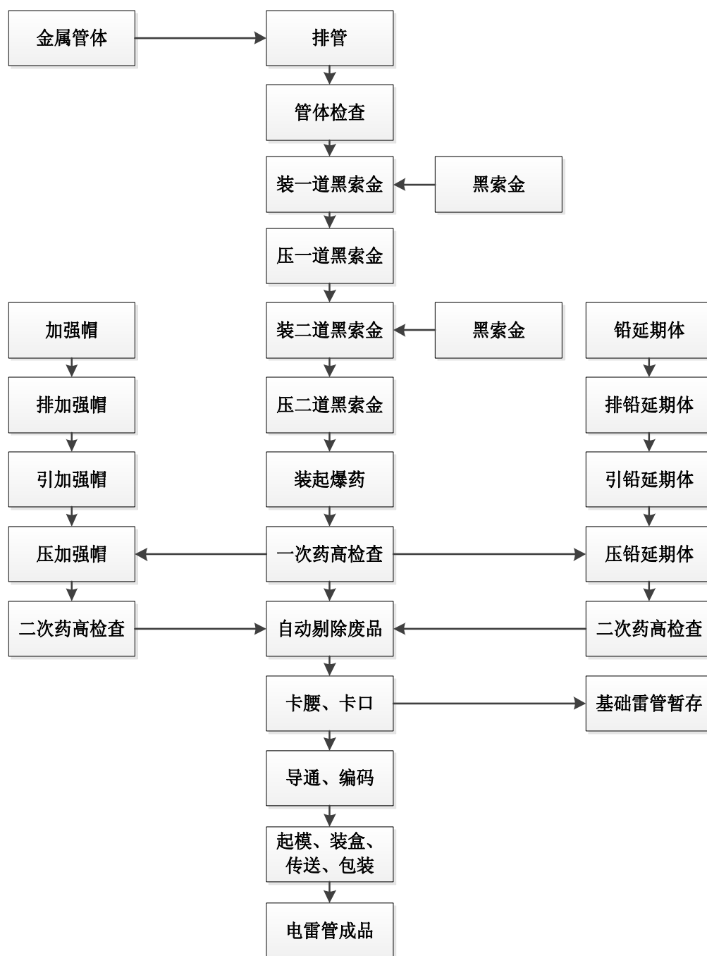
⑥导爆管工艺流程图
