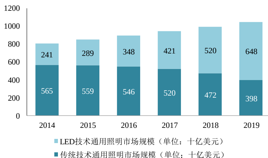
图 全球通用照明市场结构
