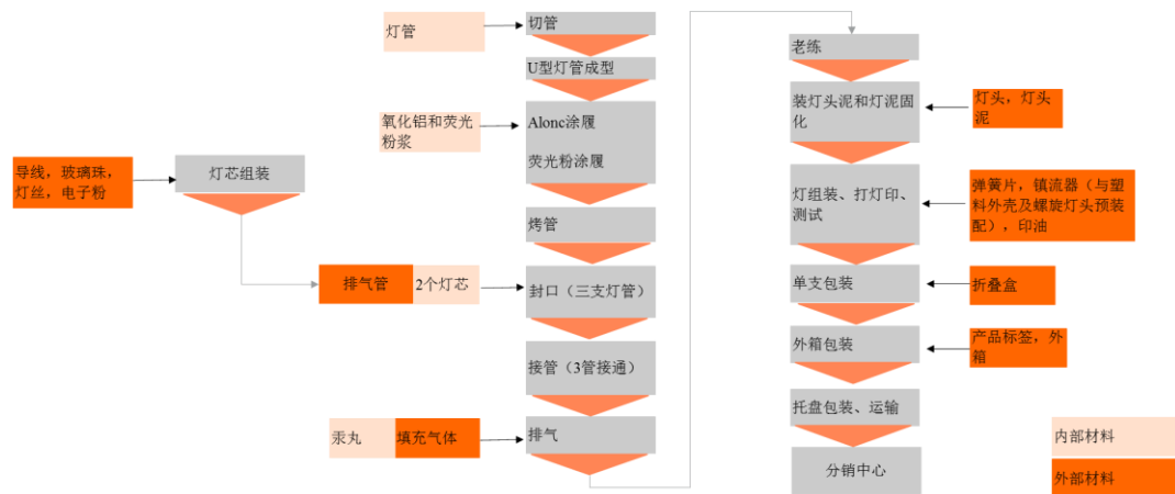
图 LPD T5/T8 核心组件工艺流程
