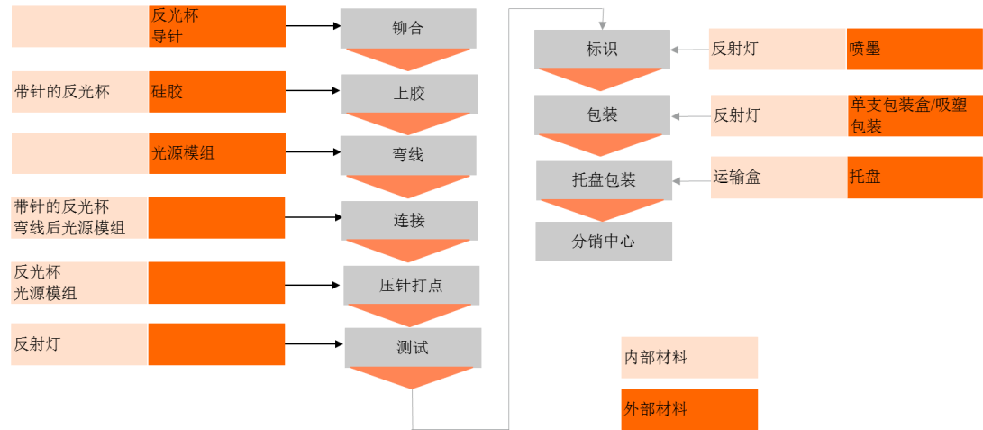
图 LED 主要产品工艺流程
