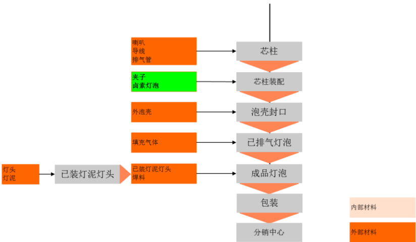
图 紧凑型荧光灯工艺流程
