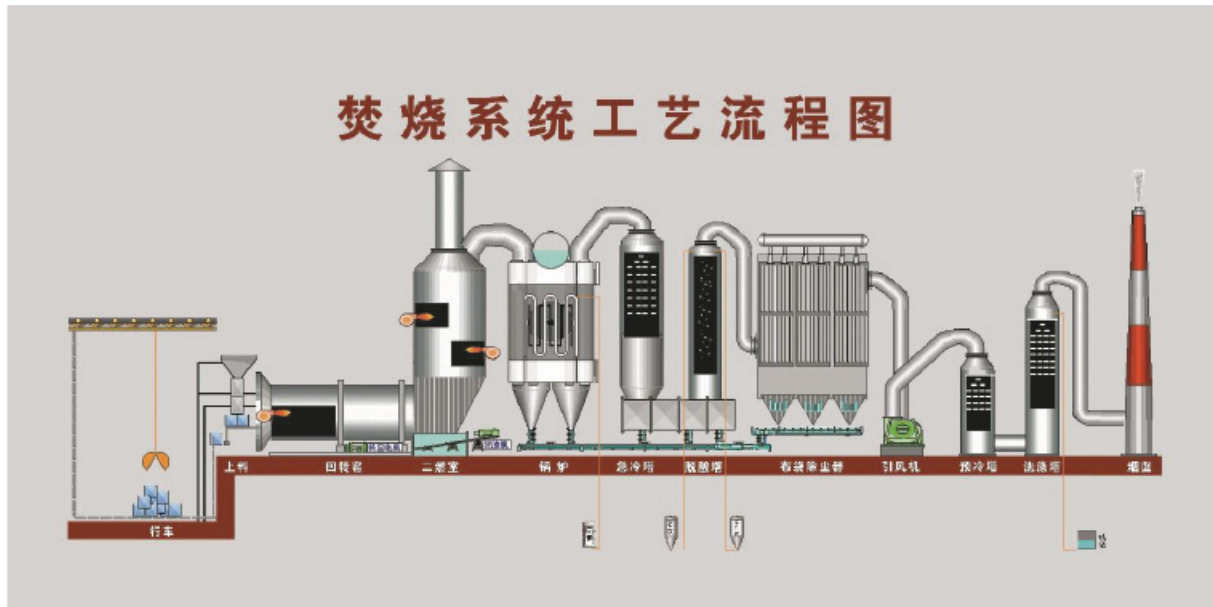
圖4.2簡化流程圖
