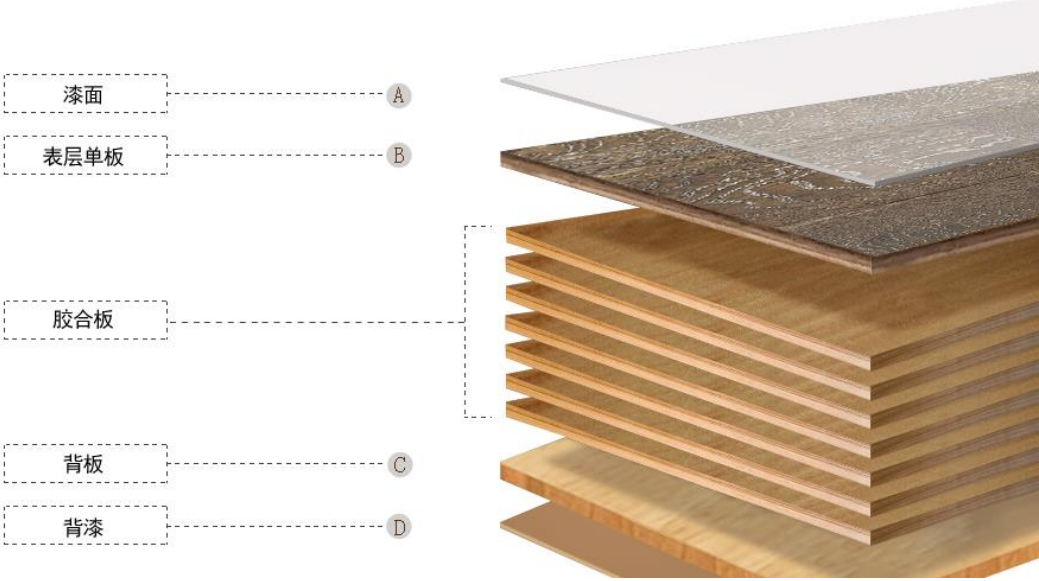
多层实木复合地板结构示意图
