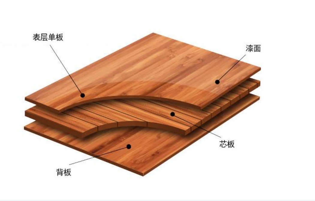
三层实木复合地板结构示意图
