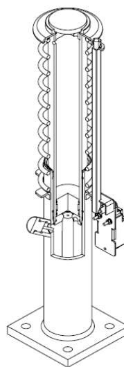
发行人缓冲器产品内部结构图示
