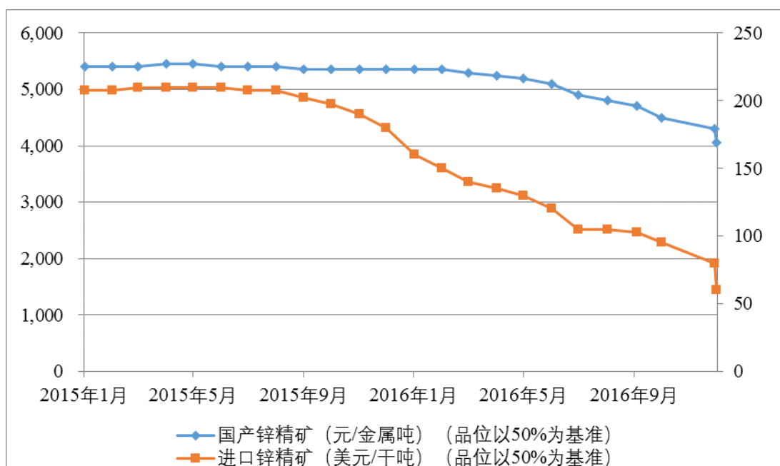
2015 年 1 月至 2016 年 12 月 锌精矿加工费的价格走势图
