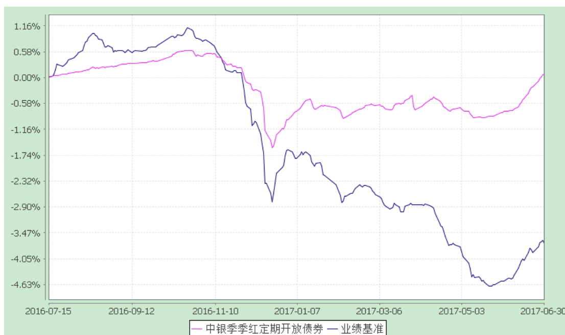
中银季季红定期开放债券型证券投资基金 累计净值增长率与业绩比较基准收益率历史走势对比图 (2016 年 7 月 15 日至 2017 年 6 月 30 日)
