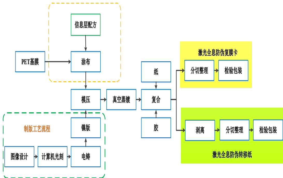
图 6-17 激光全息防伪纸生产工艺流程
