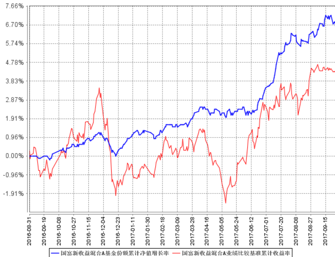
国富新收益混合A基金份额累计净值增长率与同期业绩比较基准收益率的历史走势对比图
