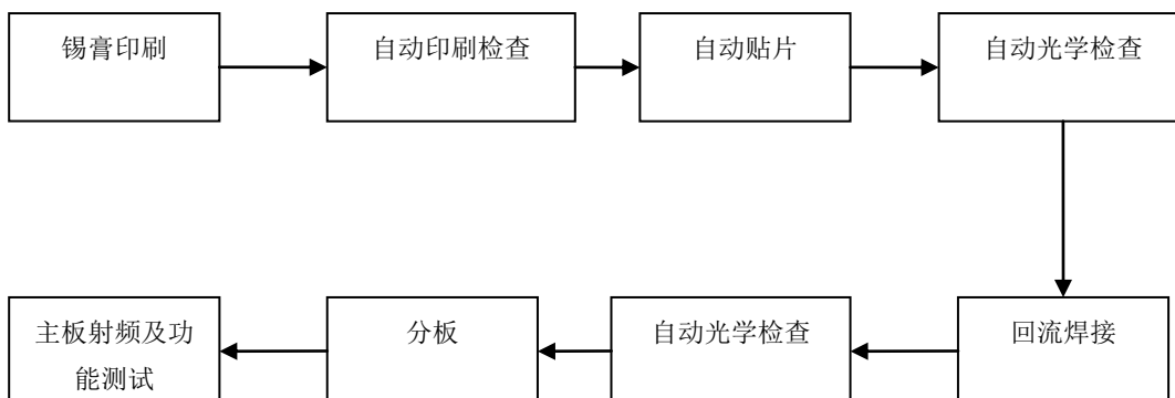
通信终端pcba(主板)工艺流程图
