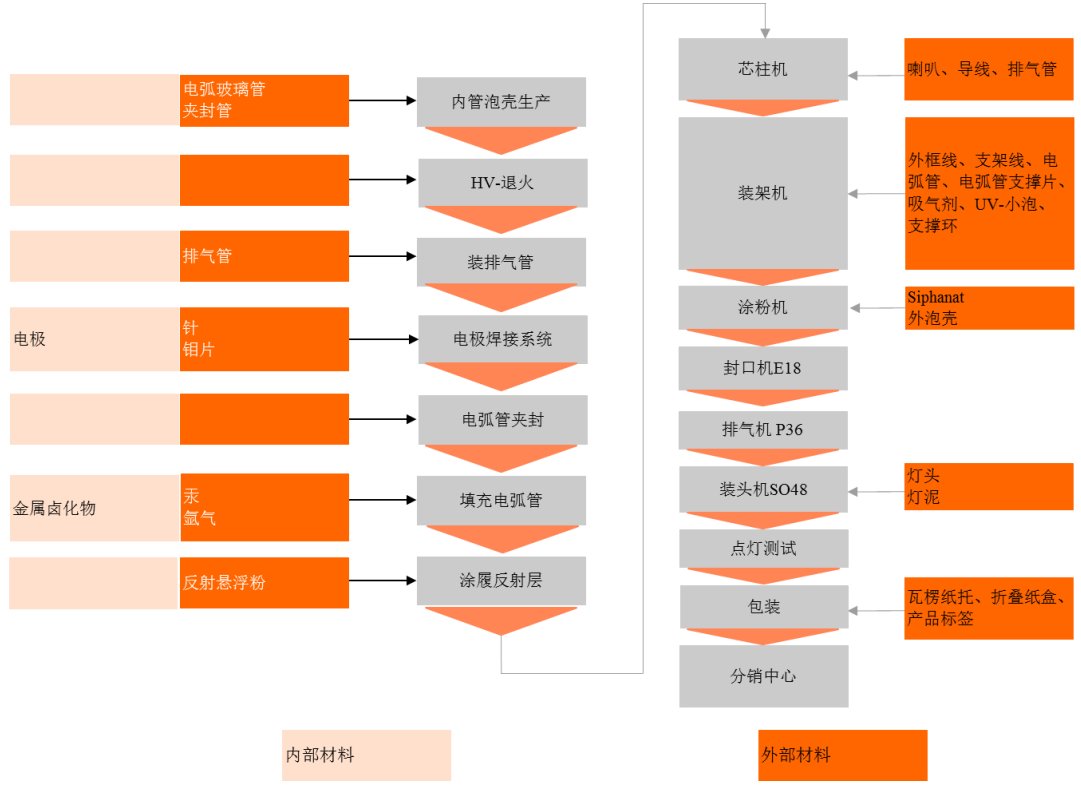
图 HPD 主要产品工艺流程
