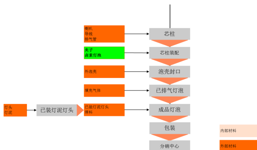
图 卤素灯工艺流程 II
