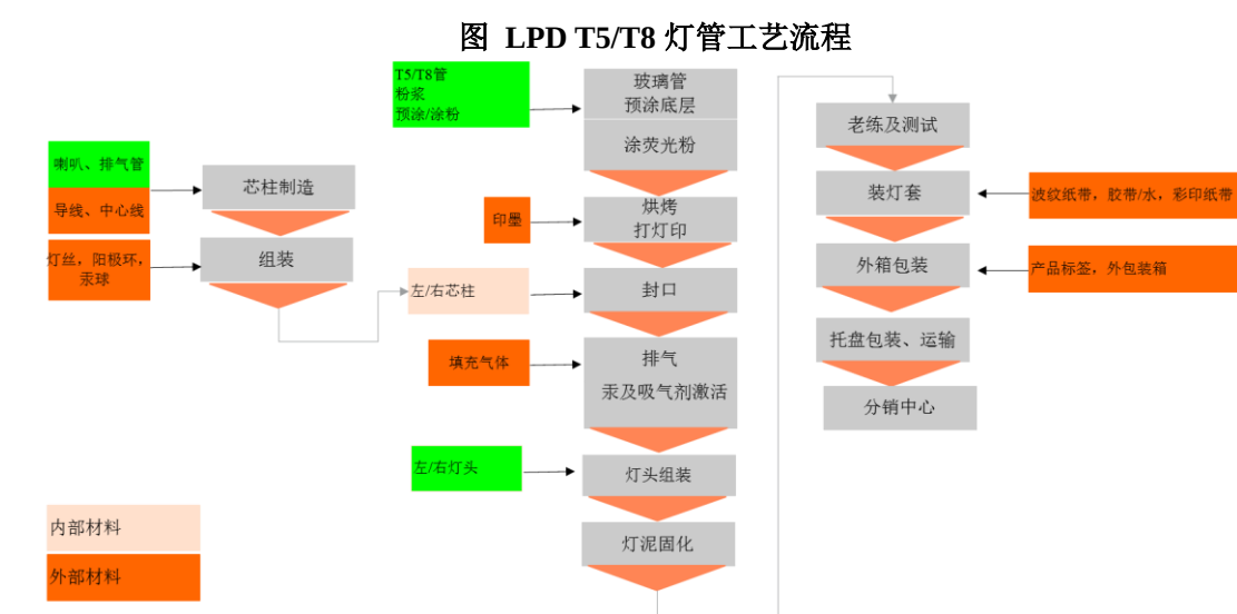
图 HPD 主要产品工艺流程
