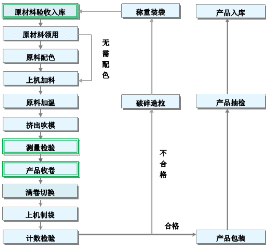
②吹膜工艺流程
