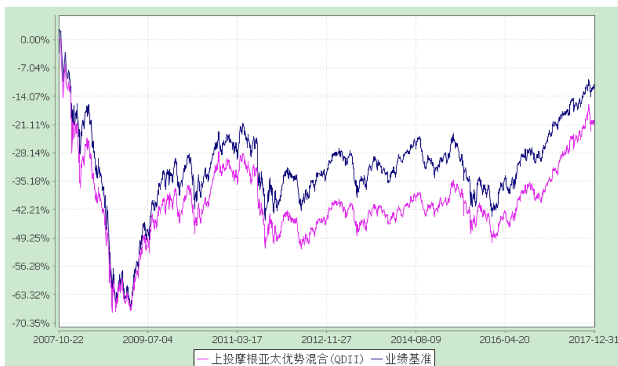
上投摩根亚太优势混合型证券投资基金 自基金合同生效以来份额累计净值增长率与业绩比较基准收益率历史走势对比图 (2007 年 10 月 22 日至 2017 年 12 月 31 日)
