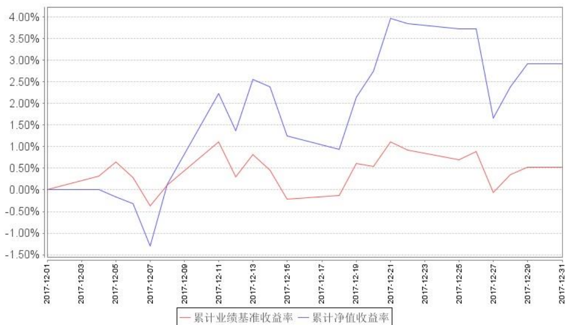
南方优选成长C累计净值增长率与同期业绩比较基准收益率的历史走势对比图
