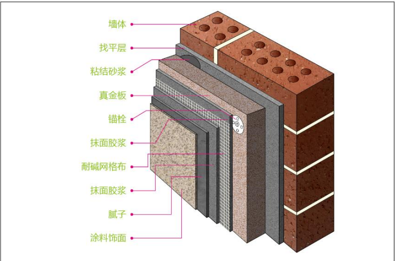
薄抹灰外墙外保温系统 构造(保温层以真金板为 例)
