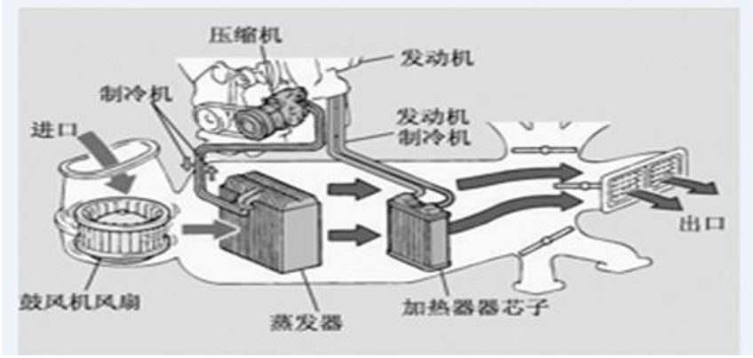
图 2-水暖式暖风系统工作原理示意图
