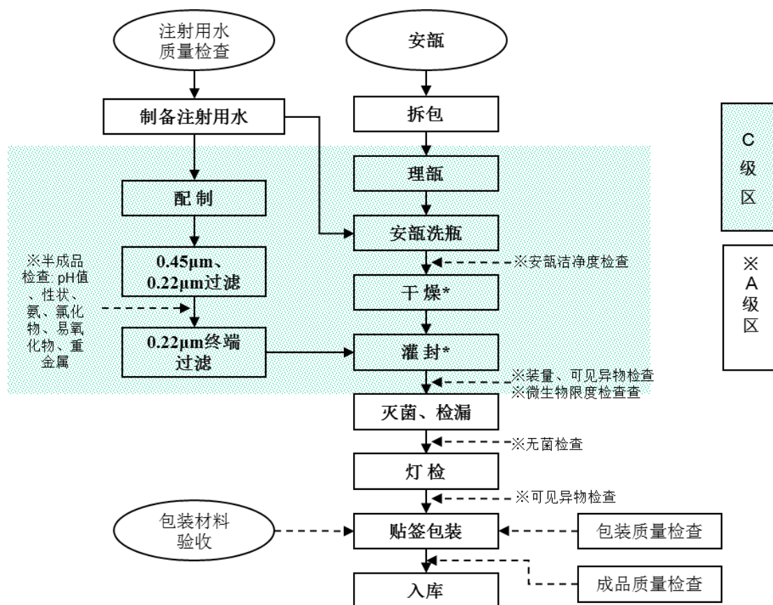
②大容量注射剂工艺流程图
