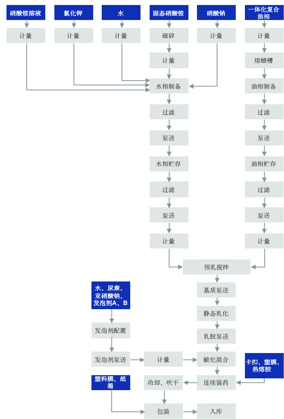
（2）改性铵油炸药生产工艺流程图：
