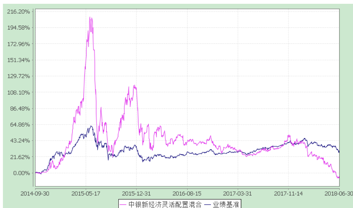
中银新经济灵活配置混合型证券投资基金 份额累计净值增长率与业绩比较基准收益率历史走势对比图 (2014年9月30日至2018年6月30日)
