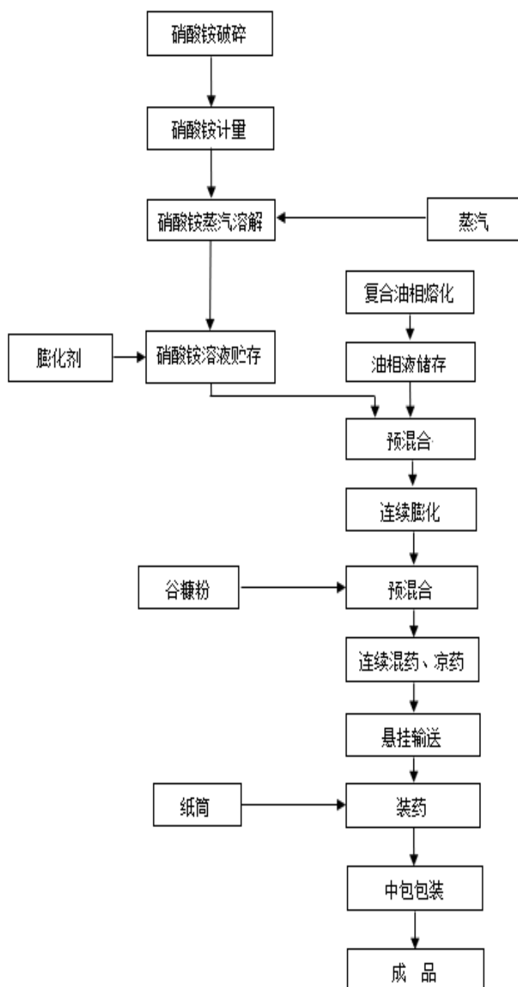
(3) 膨化硝铵炸药工艺流程图
