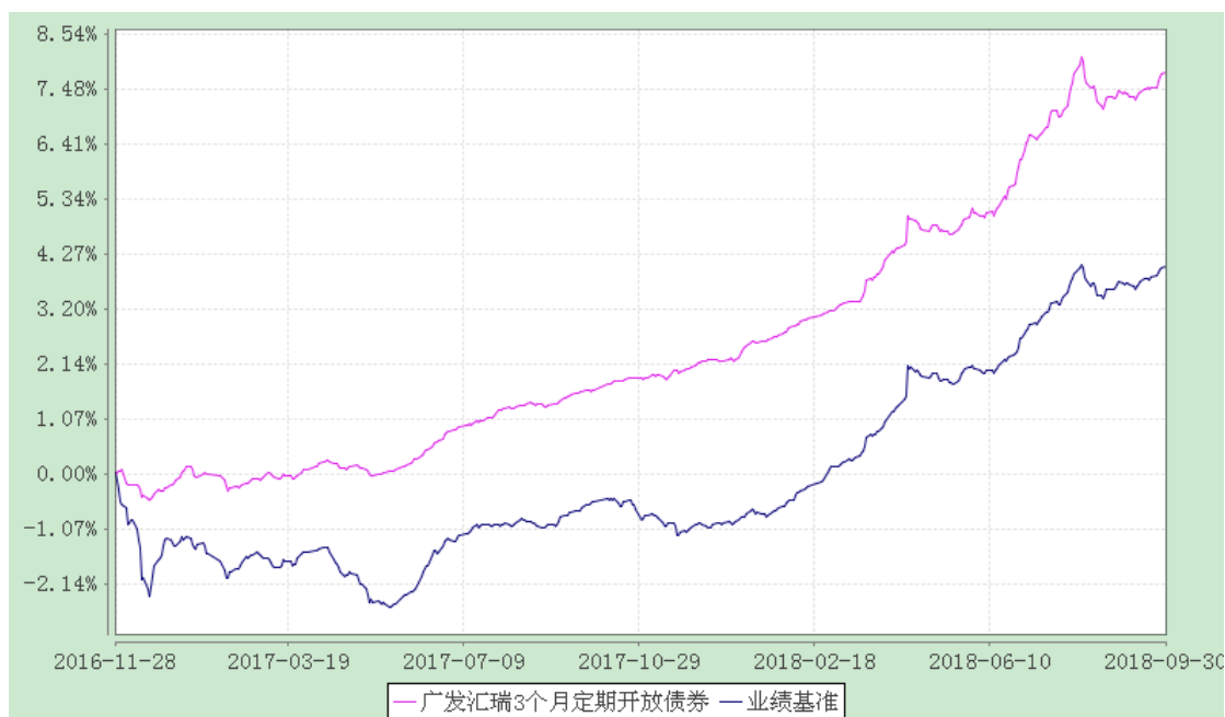
广发汇瑞 3 个月定期开放债券型发起式证券投资基金 累计净值增长率与业绩比较基准收益率历史走势对比图 (2016 年 11 月 28 日至 2018 年 9 月 30 日)
