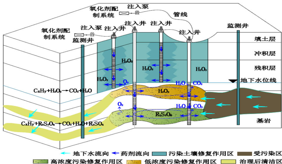
化学氧化技术工艺流程示意图
