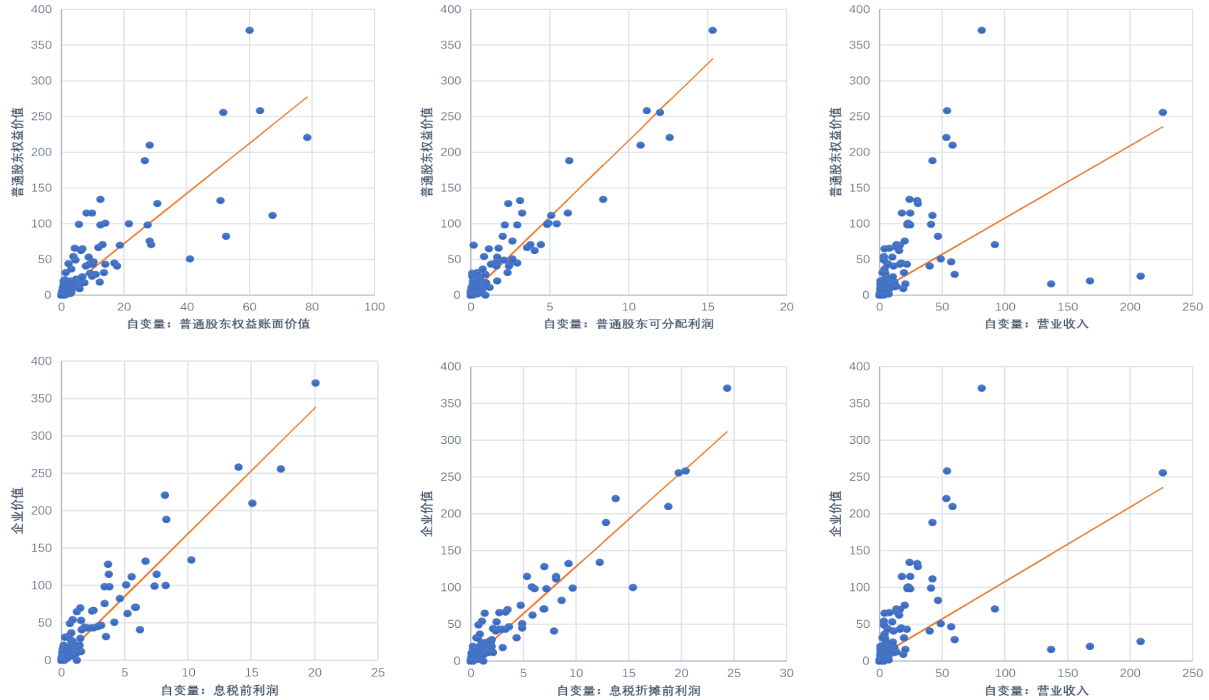
线性回归拟合图
