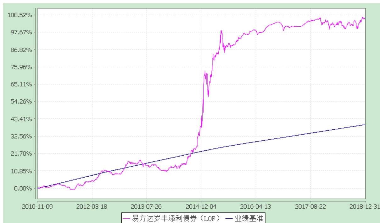
份额累计净值增长率与业绩比较基准收益率历史走势对比图 (2010 年 11 月 9 日至 2018 年 12 月 31 日)
