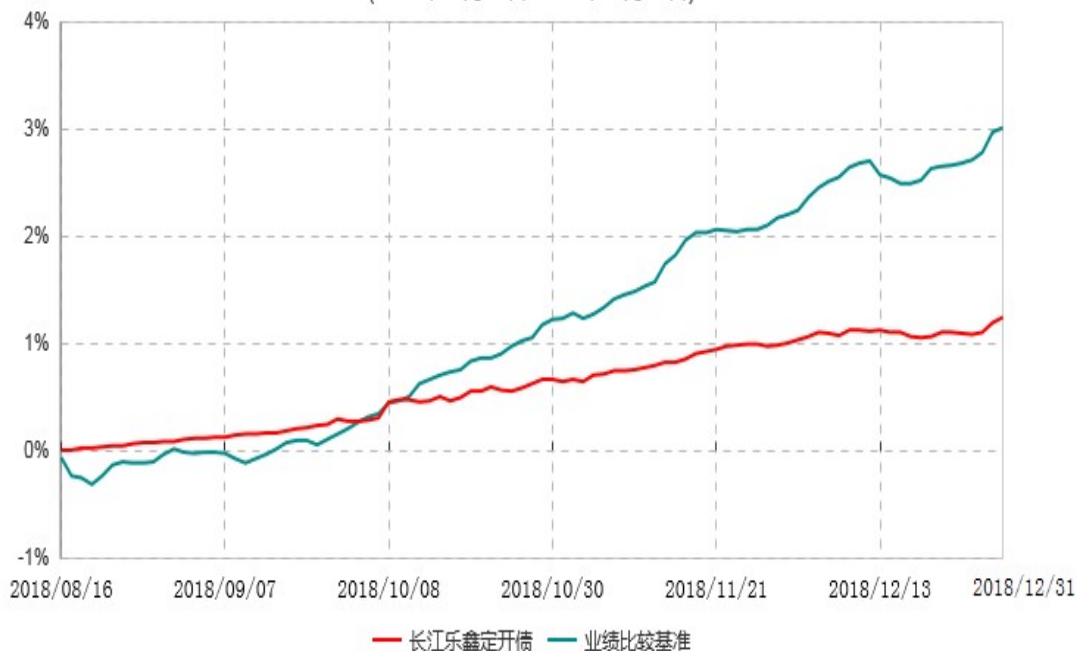
长江乐鑫纯债定期开放债券型发起式证券投资基金累计净值增长率与业绩比较基准收益率历史走势对比图
