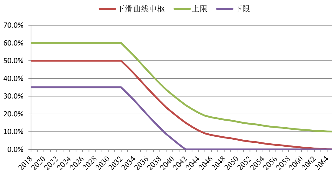
图：下滑曲线权益类资产配置比例中枢值以及权益资产投资比例上下限。
