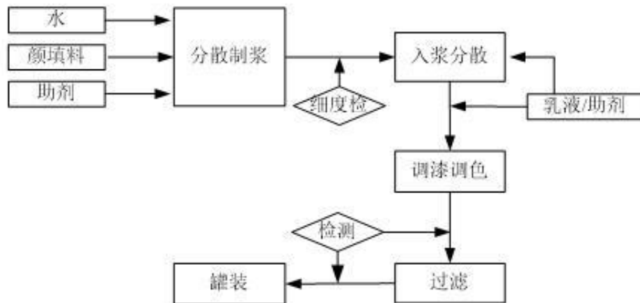
2) 木器涂料生产流程图
