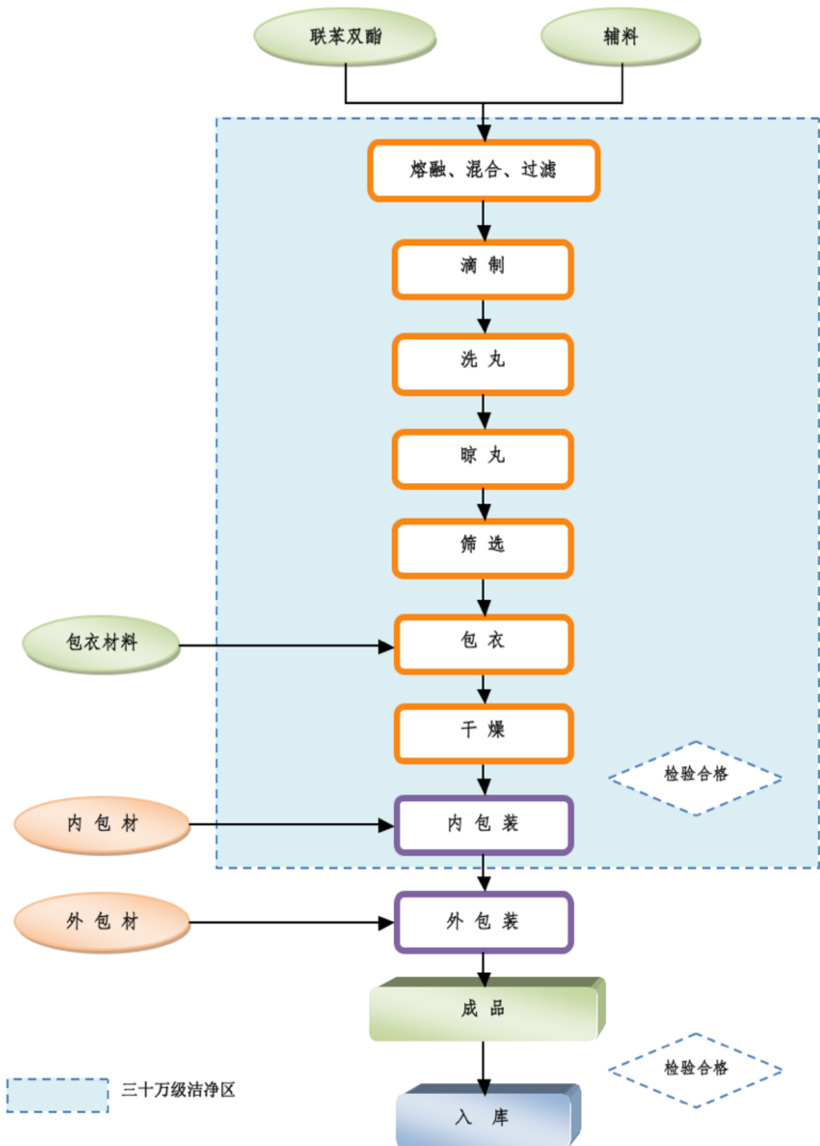
6、联苯双酯滴丸工艺流程图：
