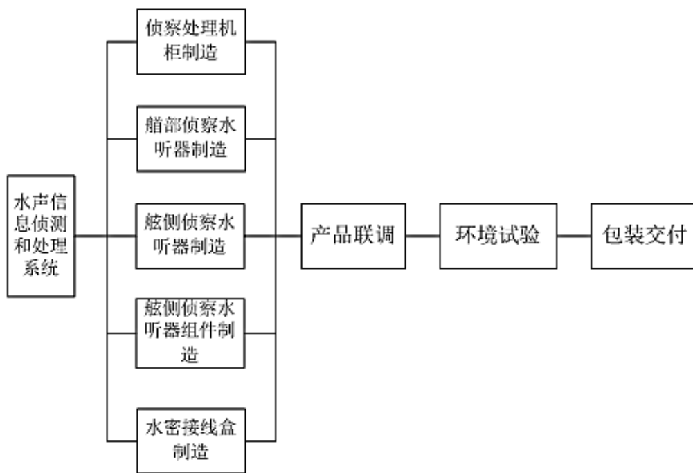
②风电配套设备主要产品生产工艺流程图
