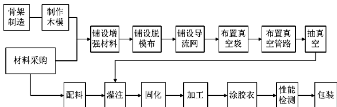
④玻璃钢制品主要产品生产工艺流程图
