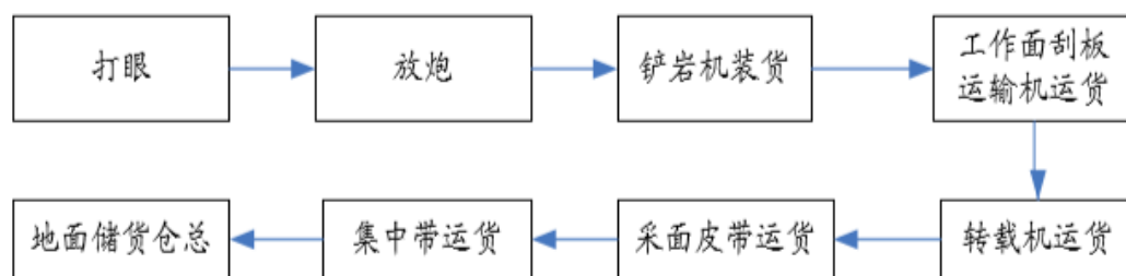
油页岩生产总工艺流程
