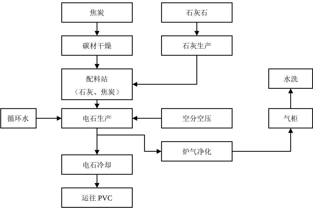
电石生产工艺流程
