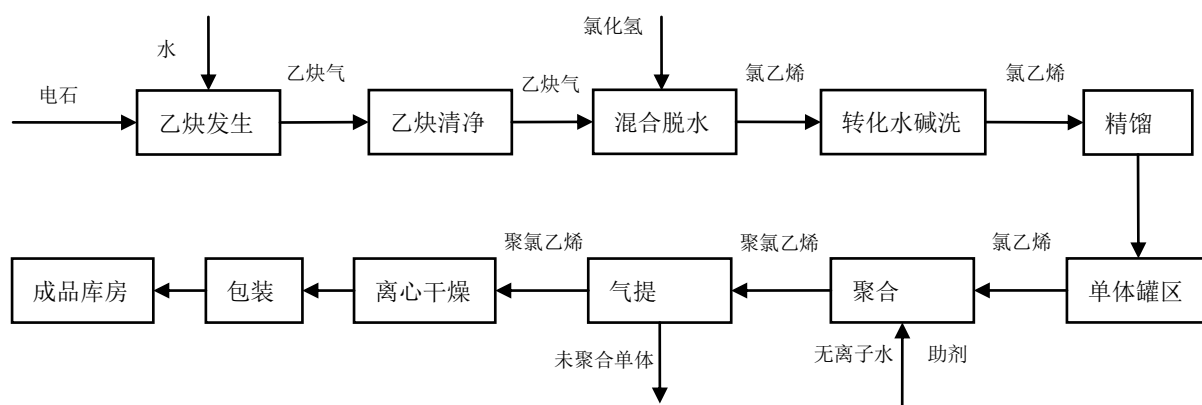
聚氯乙烯树脂产品（悬浮法）工艺流程
