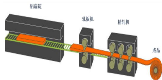
铝压延业务生产流程
