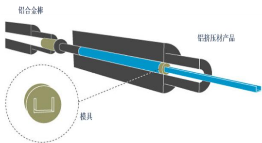
铝挤压业务生产流程
