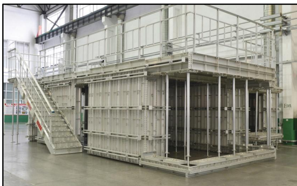
图：忠旺集团铝合金模板样板间
