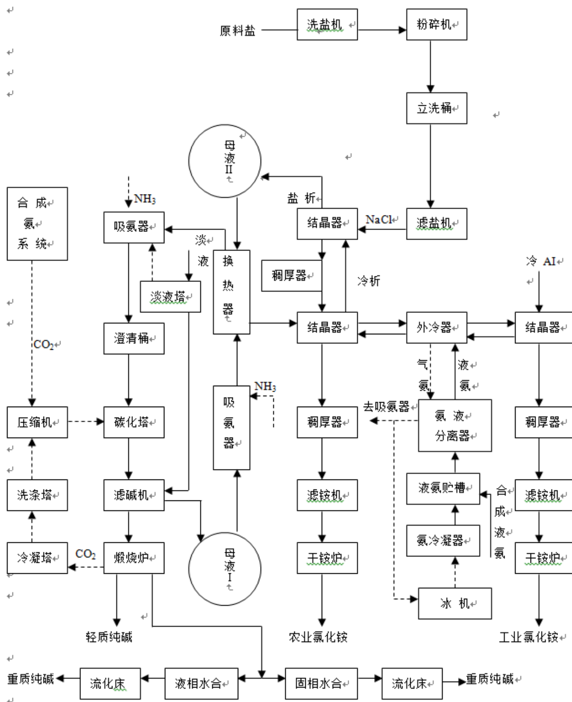
公司联合制碱法生产工艺流程图
