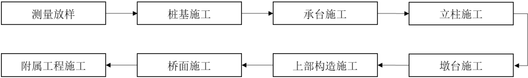
桥梁、桥涵工程施工工艺流程图如下：
