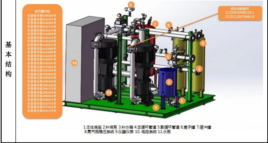
机械本体单元结构
