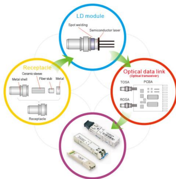
光收发接口组件、OSA 光器件在光收发模块中的应用
