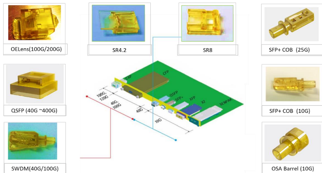
光纤阵列透镜- Lens Array
