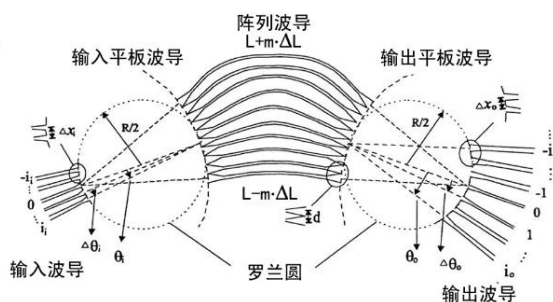
AWG 的结构与原理
