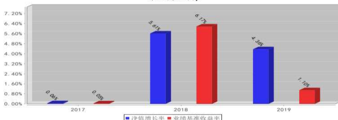
泰达宏利交利债券 C 基金每年净值增长率与同期业绩比较基准收益率的对比图(2019 年 12 月 31 日)
